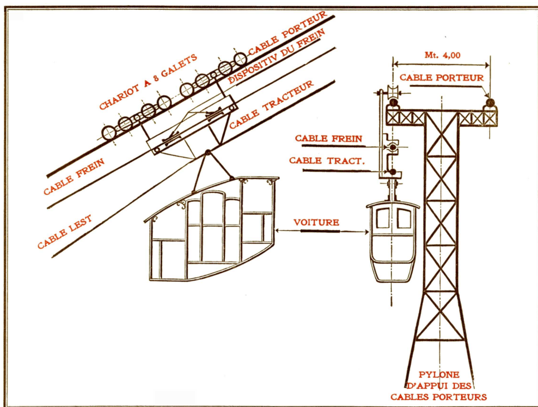
ELEVATION SCHEMATIQUE DU CHARIOT AVEC VOITURE ET PYLON.
