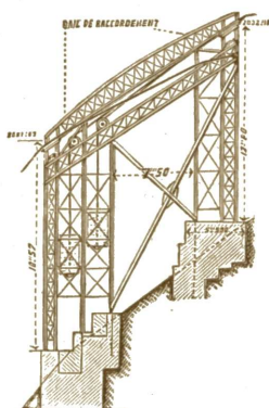
DISPOSITIF INTERMEDIAIRE DE TENSION DES CABLES PORTEURS.
